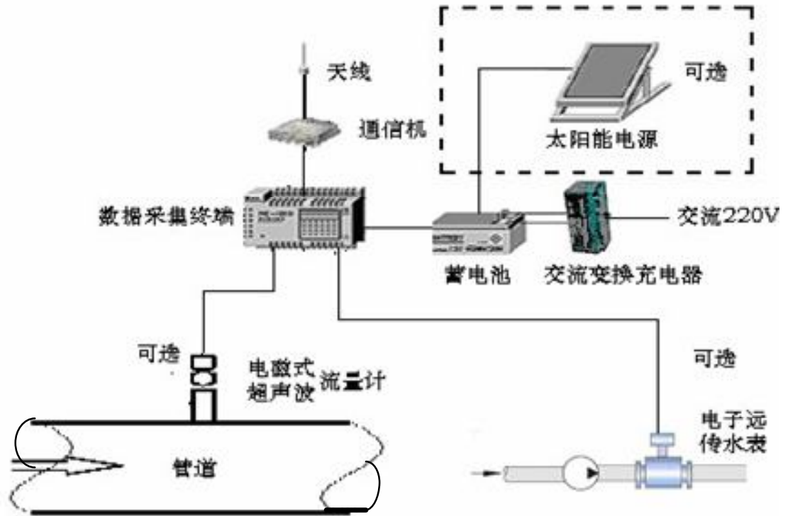
图6 管道流量自动监测站结构图
