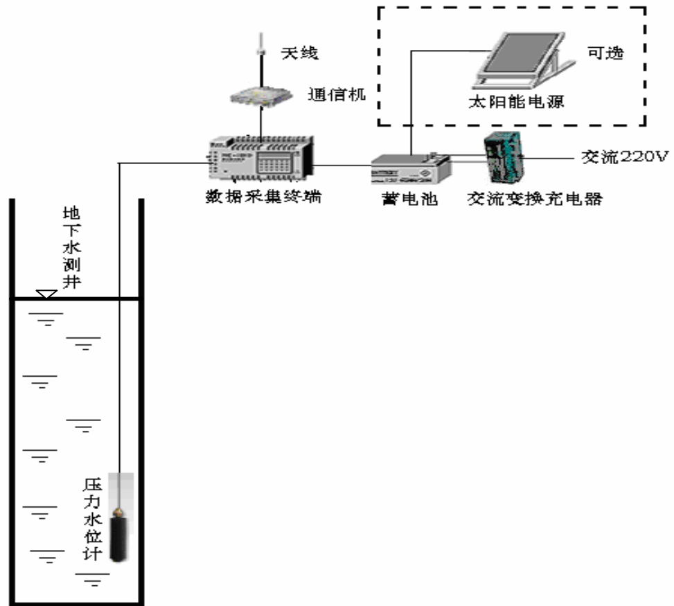
图7 地下水自动监测站结构图
