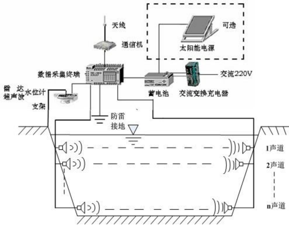
图1 超声波时差法监测站结构图
