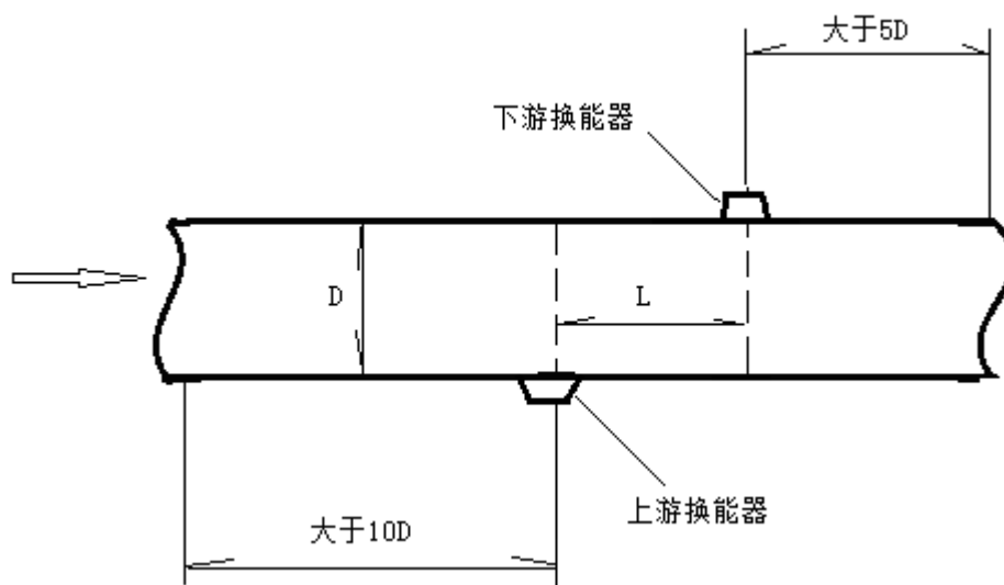
图18 Z方式安装换能器
