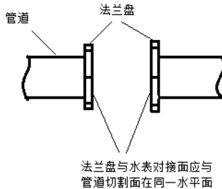
图12 法兰盘安装要求
