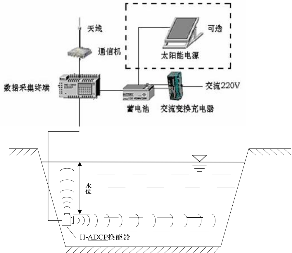
图2 水平式声学多普勒流速仪监测站结构图
