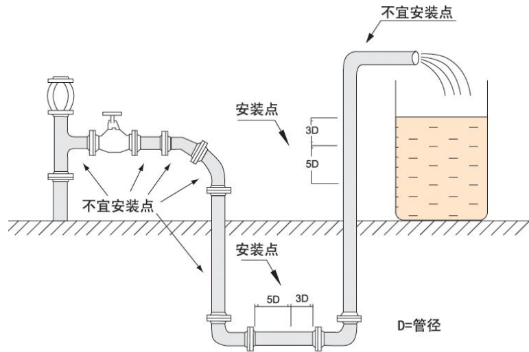
图 13-2 电磁式管道流量计安装位置图
