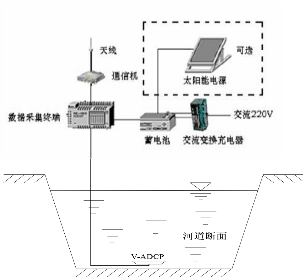
图3 座底式声学多普勒明渠流量计监测站结构图
