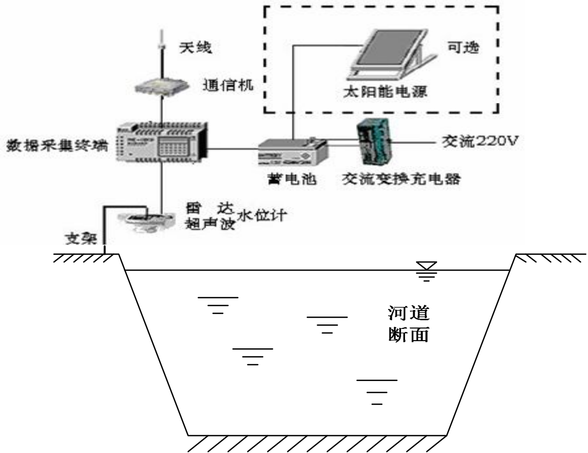
图4 水位监测站结构图
