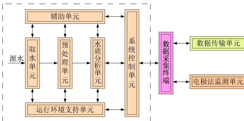
图8 水质自动监测站结构图
