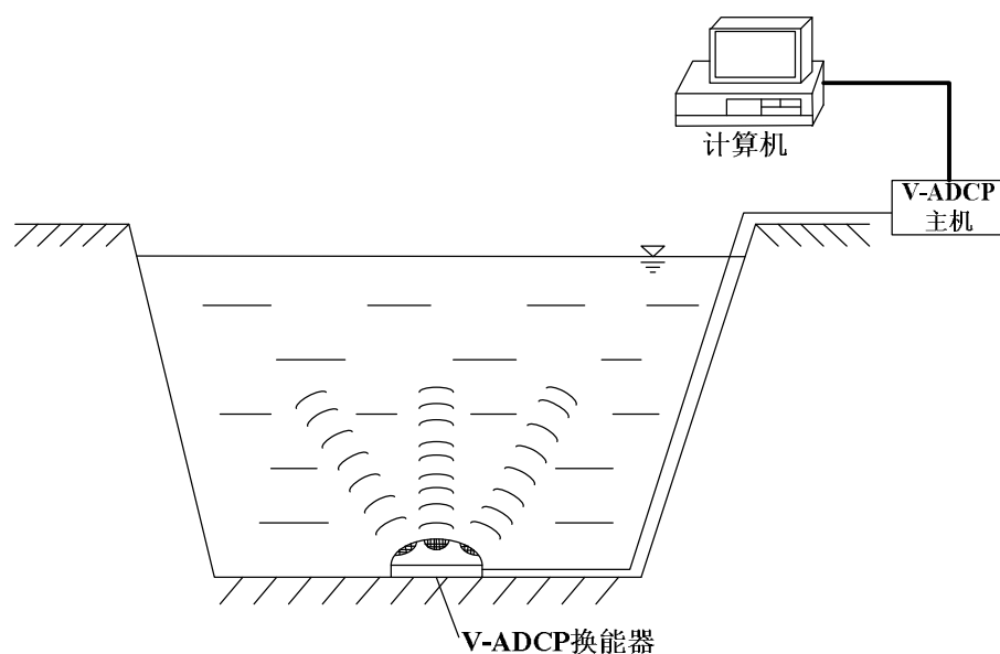
图11 V-ADCP 主机安装示意图
