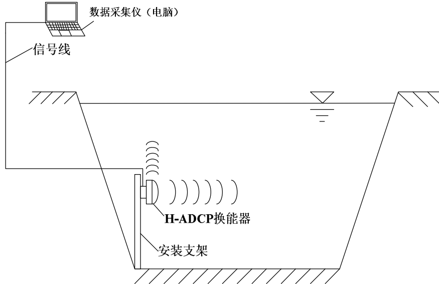
图10 H-ADCP 主机安装示意图
