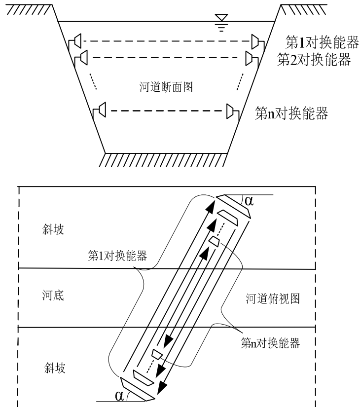
图9 换能器安装示意图
